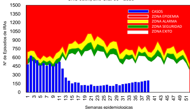
Canal Endémico de IRAs por Semana Epidemiológica SRS Jaén, año S.E. 39 - 2020
